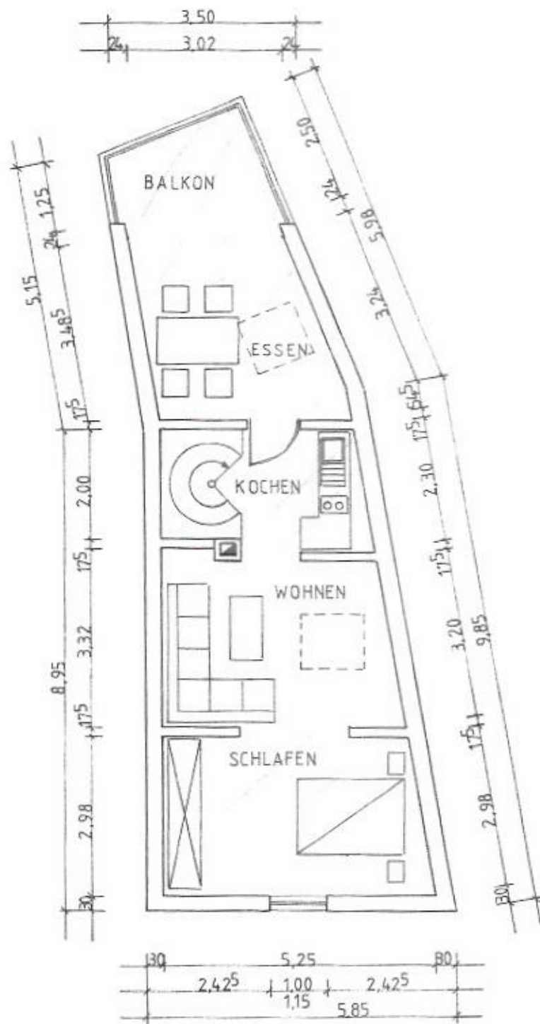
GRUNDRISS DACHGESCHOSS (KNIESTOCK) M 1:100
