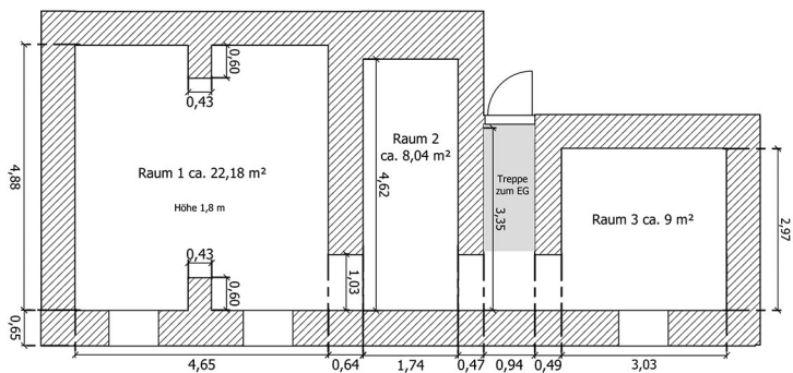
Keller (teilunterkellert)
