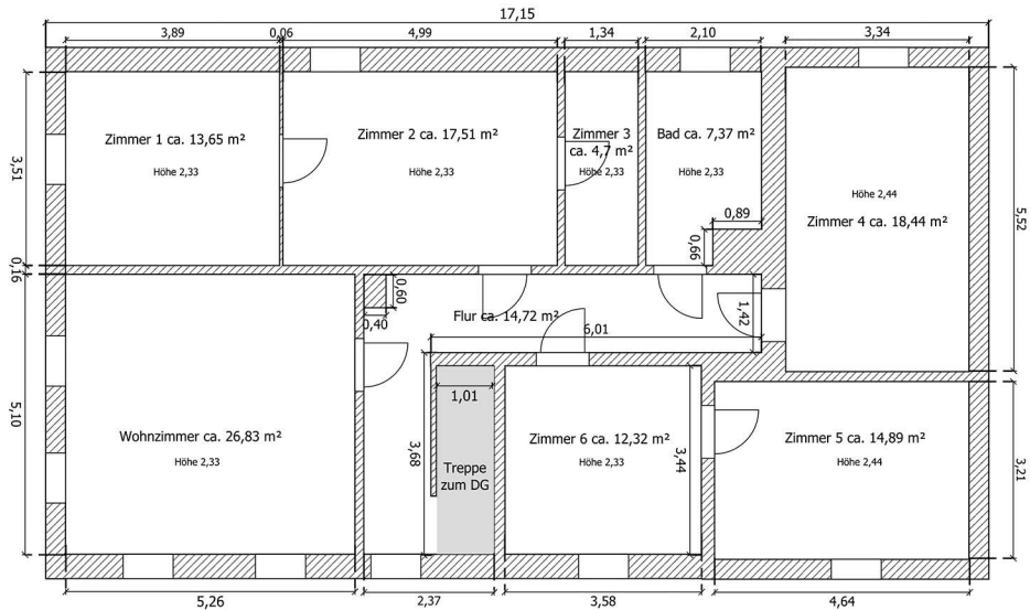
großes Wohnhaus - Obergeschoss
