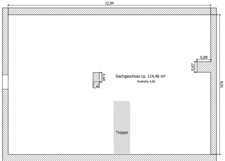
großes Wohnhaus - Dachgeschoss
