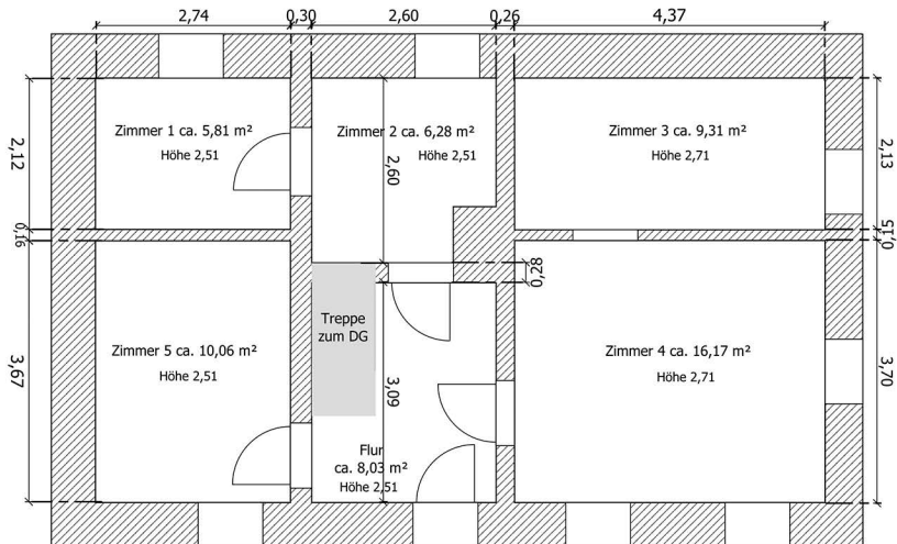
Erdgeschoss - kleines Wohnhaus
