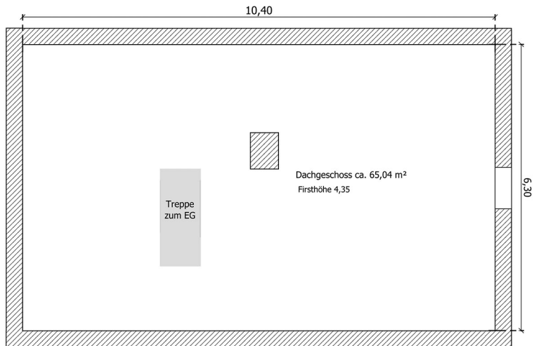
Dachgeschoss - kleines Wohnhaus
